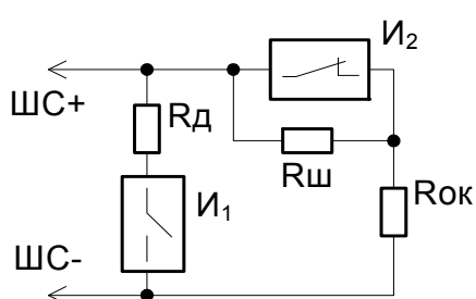
Рисунок 5. Схема подключения дымовых и тепловых извещателей в шлейфы типа 2
