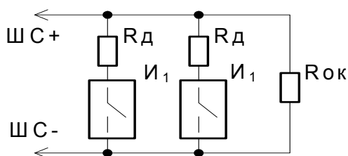
Рисунок 4. Схема подключения дымовых извещателей в шлейфы типа 1
