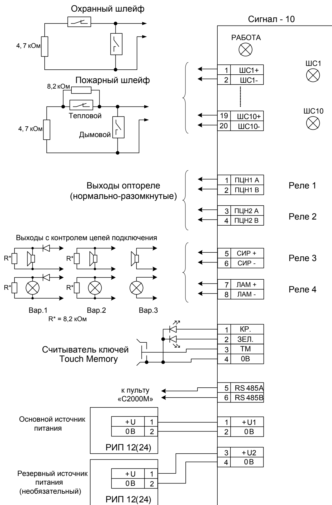
Рисунок 3. Схема подключений прибора Сигнал-10 при эксплуатации
