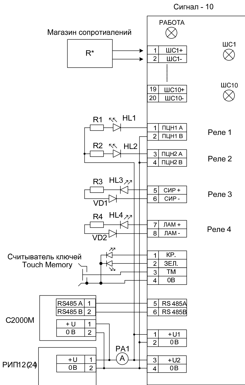
Рисунок 18. Схема подключения прибора Сигнал-10 при общей проверке
