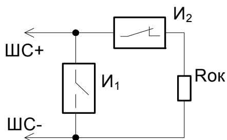
Рисунок 7. Схема подключения охранных извещателей в шлейф типа 5
