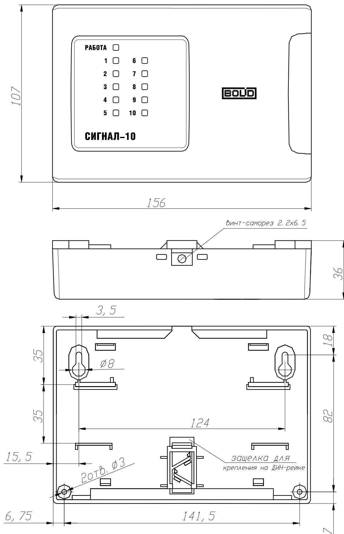
Рисунок 2. Габаритные и установочные размеры прибора Сигнал-10
