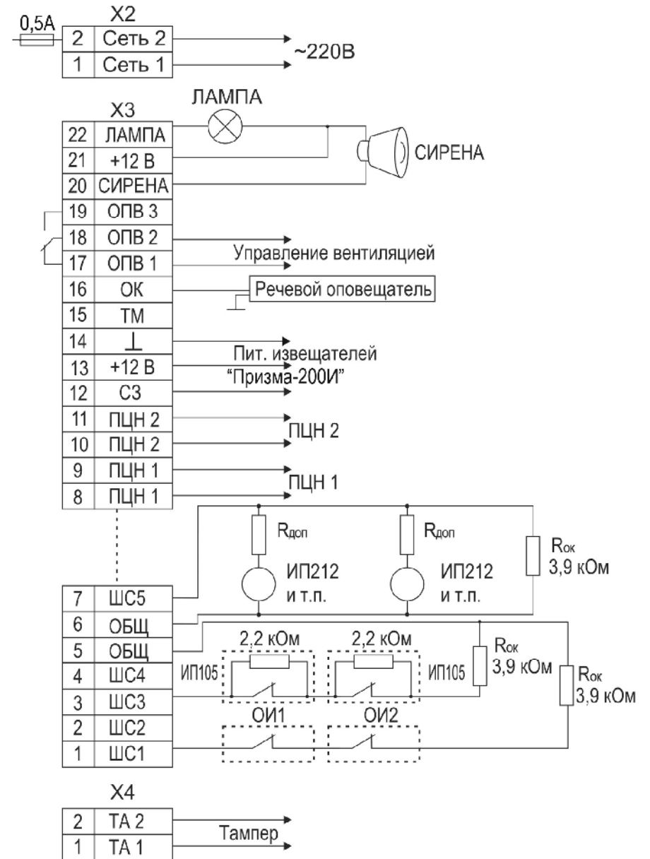
Рис.2. Схема внешних соединений "Гранит-5"
